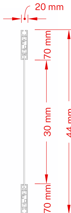
Sezione fronte
